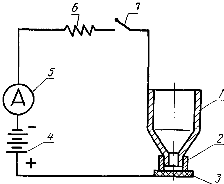
Схема установки
