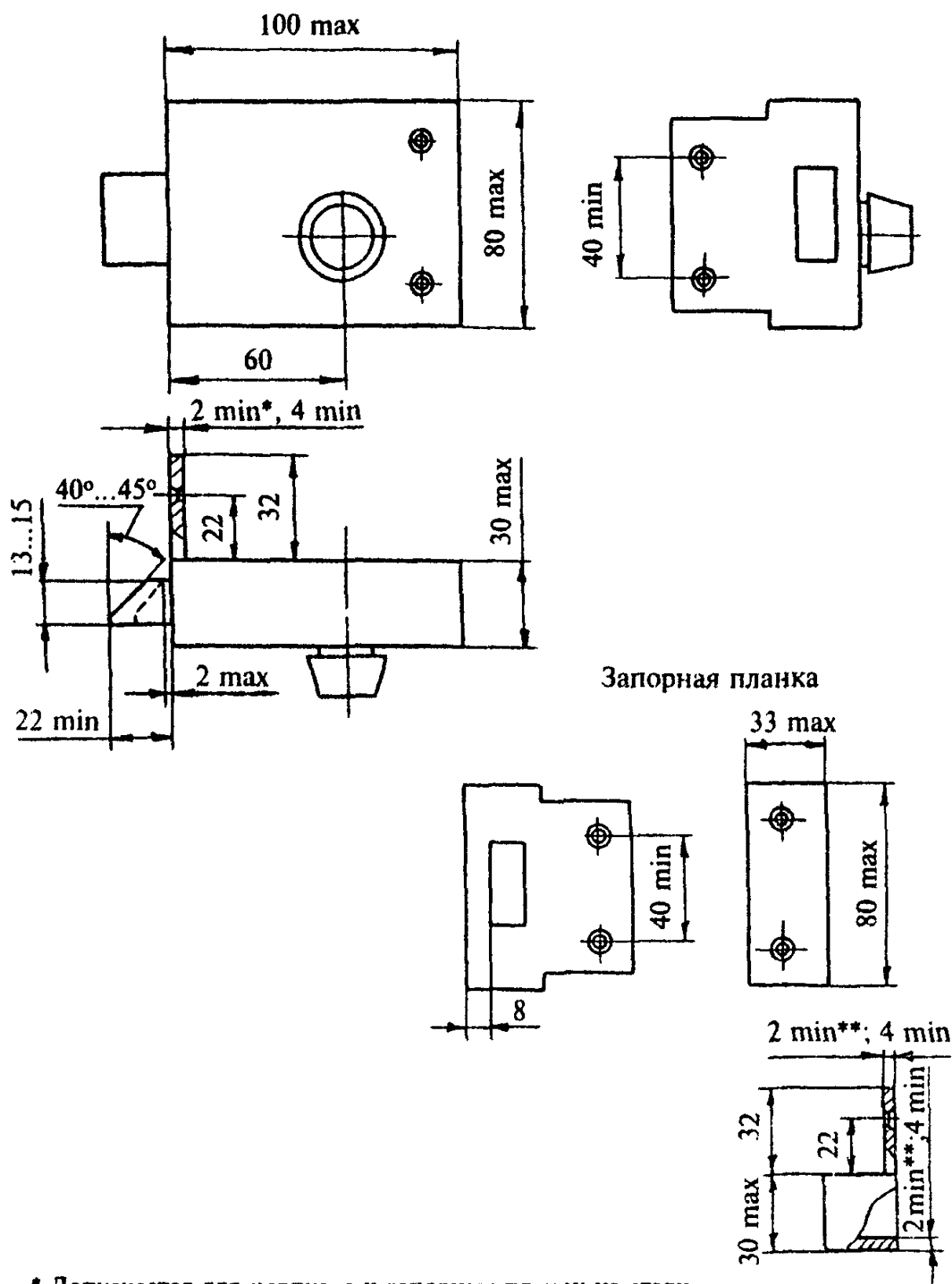
Рисунок А.7 — Замок накладной, тип ЗН2
