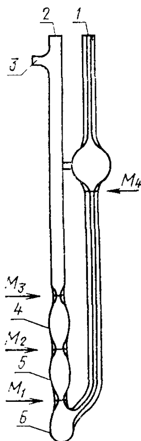
Вискозиметр типа ВНЖТ (Канон-Фенске- Опакв)
