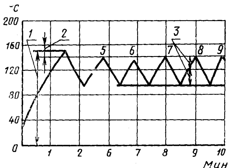
Диаграмма измерения температуры подошвы утюга
