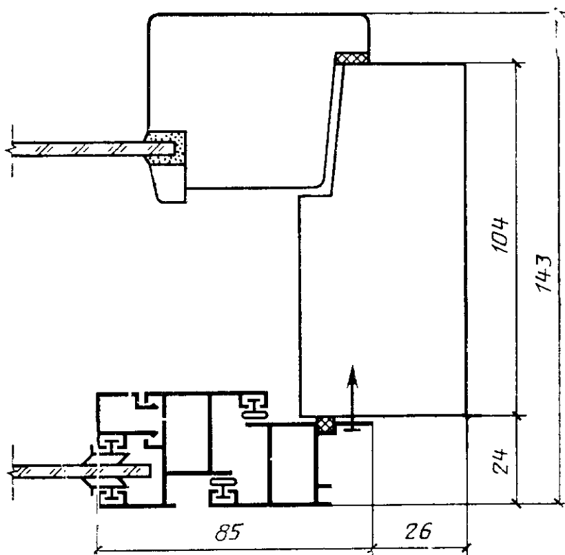
Сечение 4
