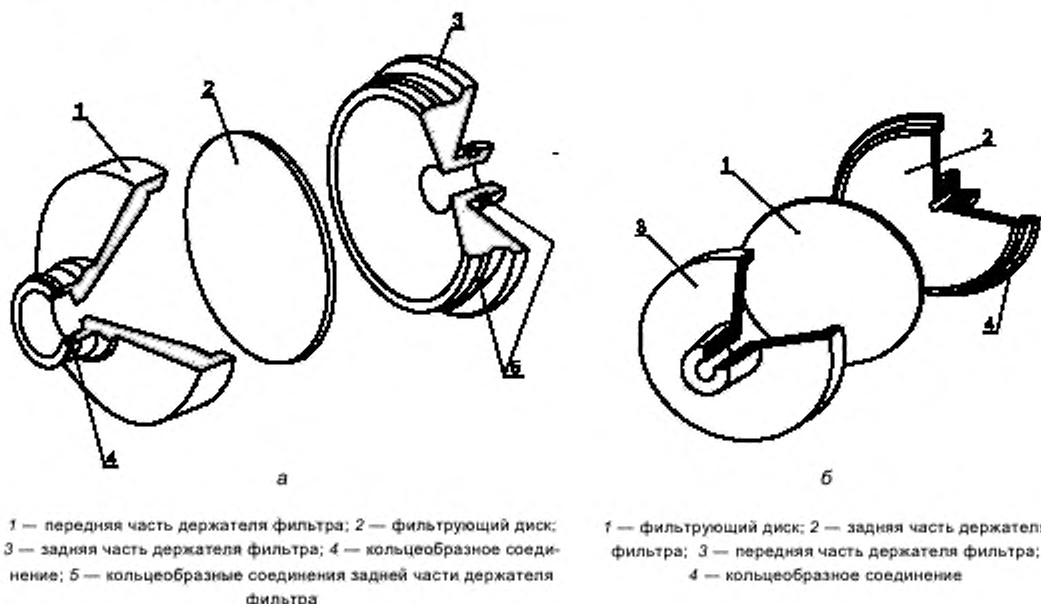
Рисунок 4 — Схема ловушки для дыма с фильтрующим диском из стекловолна
