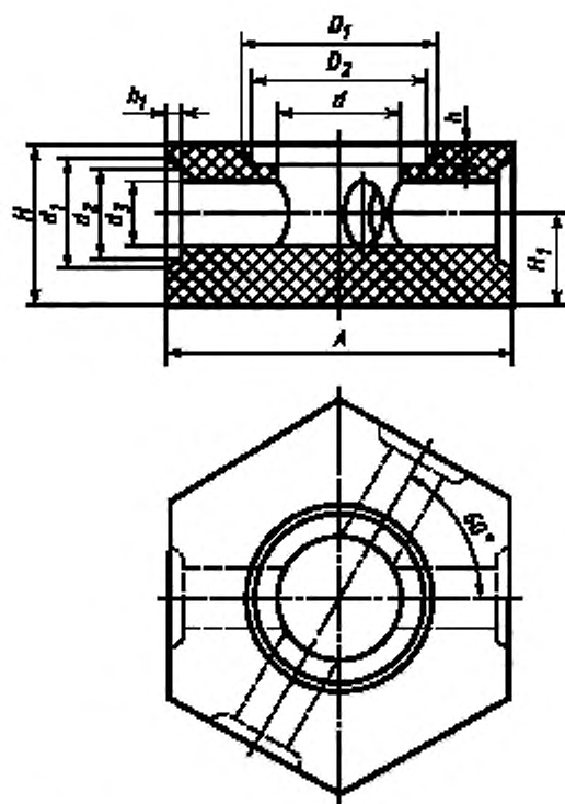
Рисунок 7 — Косоугольная четырехходовая звездочка с лазером
