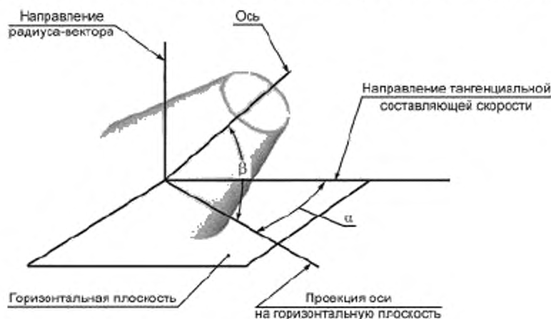
Рисунок 7.2 — Задание ориентации элемента конструкции КА
