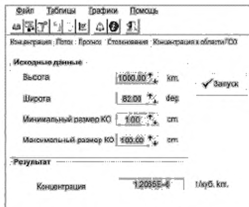
Рисунок А.2 — Панель пункта меню «Концентрация»
