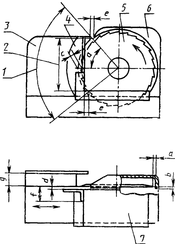
1—рабочее отверстие; 2—полная высота рабочего отверстия; 3—пластина, регулирующая толщину нарезаемых ломтей; 4—защита большого пальца; 5—нож; 6—защита ножа; 7—подающая доска; g—толщина ломтя.
