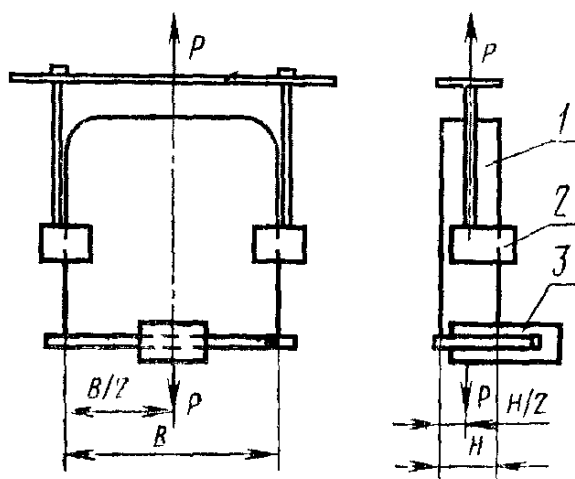
1—ящик (полуящик); 2—приспособление; 3—захват машины.
