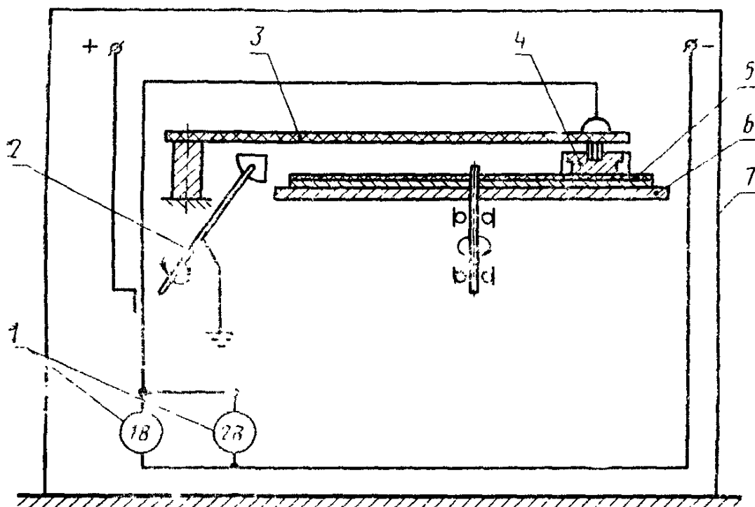
1—килвольтметры; 2—заземленный поворотный рычаг; 3—подвижный рычаг; 4—головка; 5—кассета с образцом; 6—диск; 7—камера
