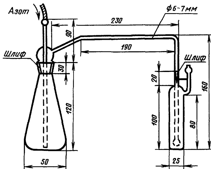
Прибор для отгонки сероводорода
