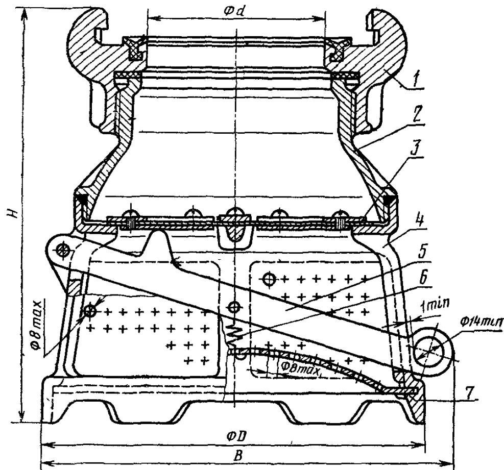
Типоразмер СВ-125
