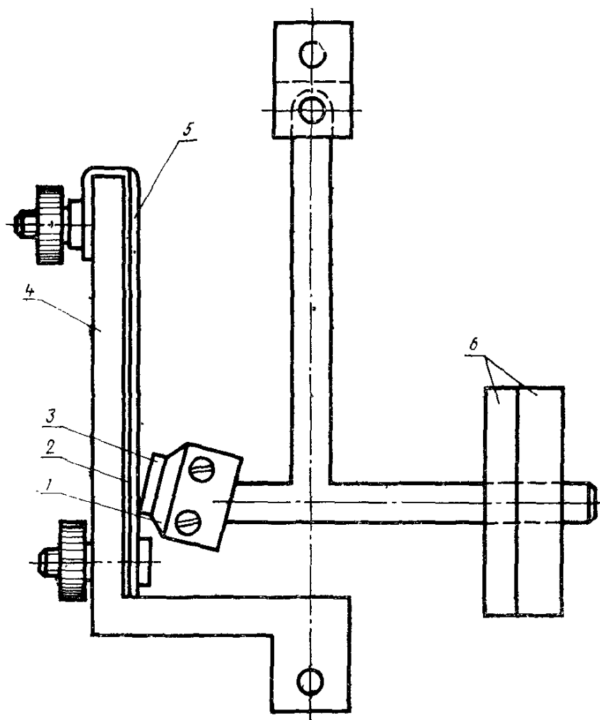
Схема приспособления на порез к разрывной машине
