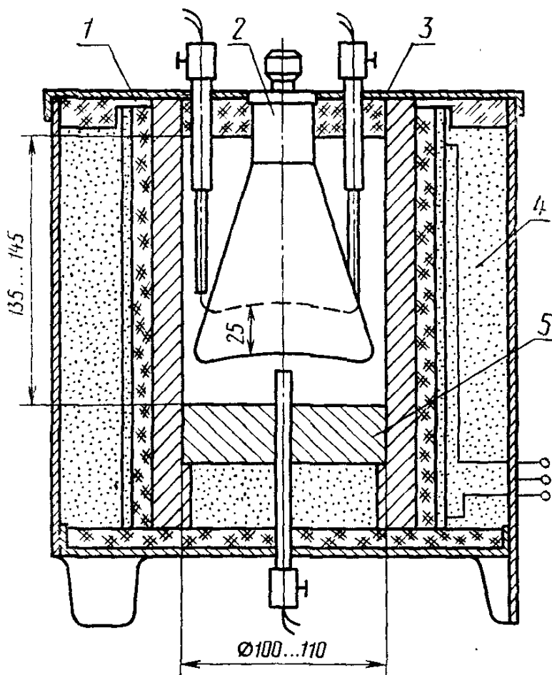
1—огнеупорный цилиндр; 2—колба; 3— крышка; 4—металлический цилиндр; 5— вставка
