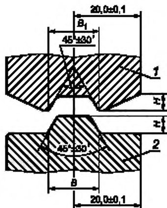
1 — муфта с выемкой; 2 — муфта с выступом
