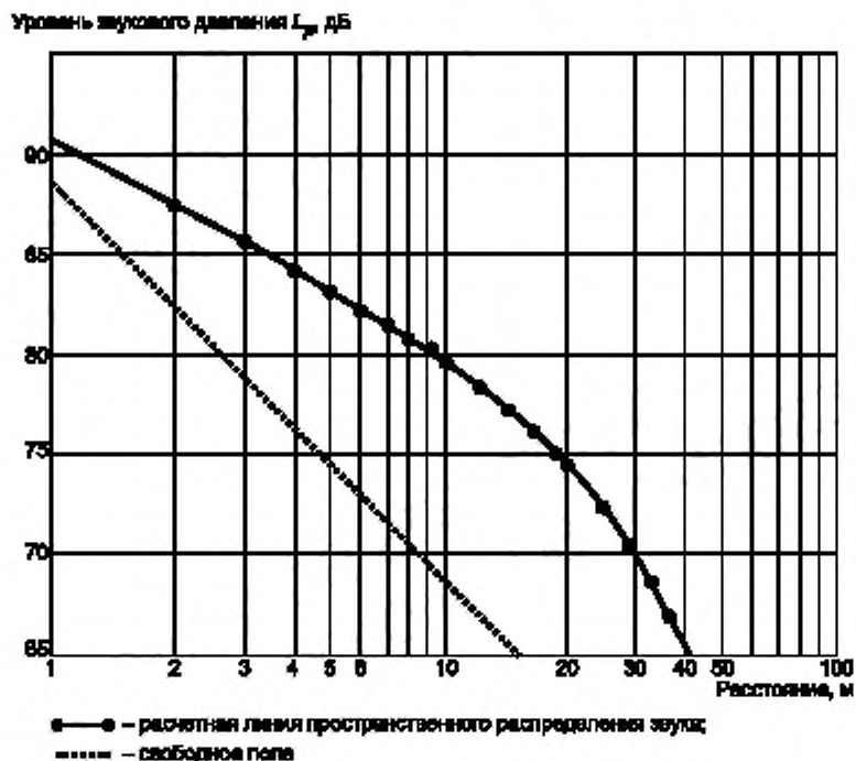
Рисунок А.4 — Рассчитанная линия пространственного распределения звука. Уровень звуковой мощности источника равен 100 дБ
