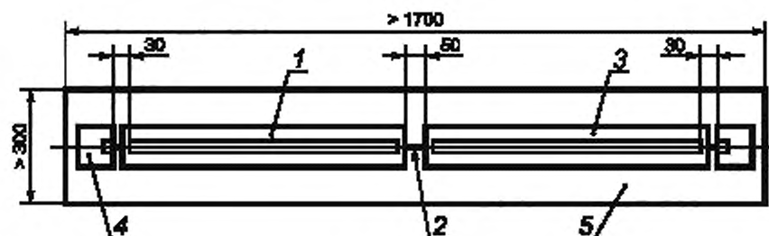
Рисунок Б.4 — Фиксирующее устройство для калибровки (вид сверху)
