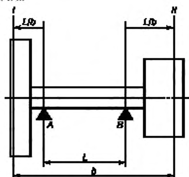
А, В — плоскости задания допуска (плоскости подшипников); I, II — плоскости коррекции
