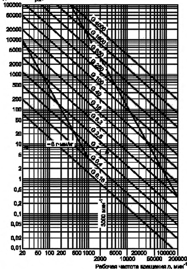
Рисунок А.2 — Пример определения e_{per} с помощью рисунка 2
