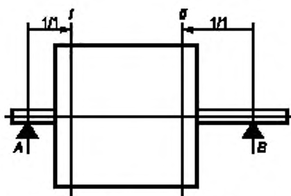
А, В — плоскости задания допуска (плоскости подшипников); I, II — плоскости коррекции
