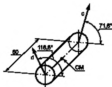
д) Векторы дисбалансов в торцевых плоскостях ротора
