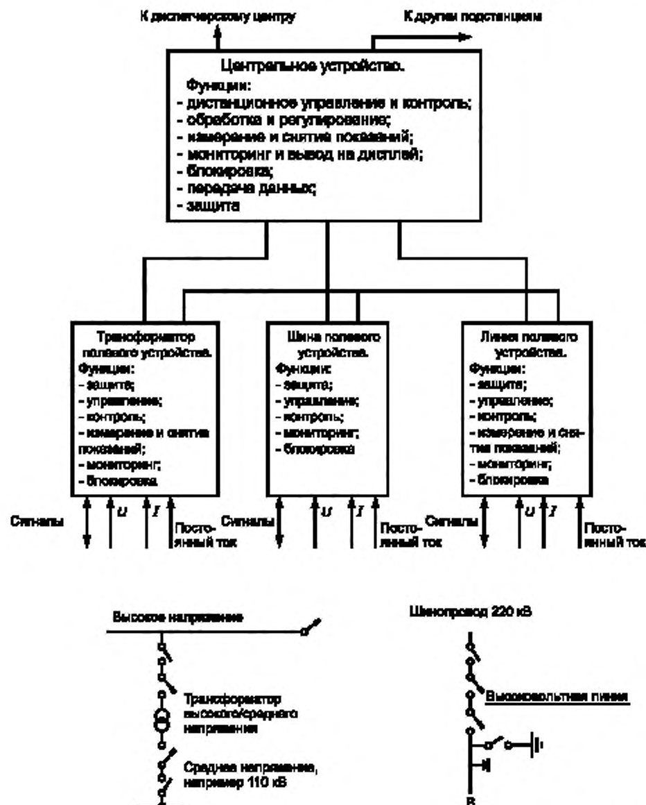
Рисунок Б.5 — Общая структура системы контроля и управления высоковольтной подстанции
