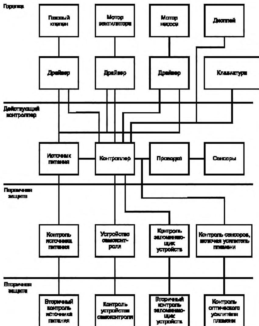
Рисунок Б.3 — Контроллер газовой горелки: блок-схема
