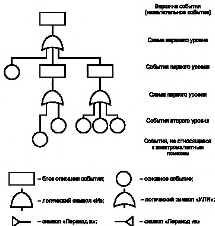
Рисунок Б.1 — Символы для конструирования дерева неисправностей
