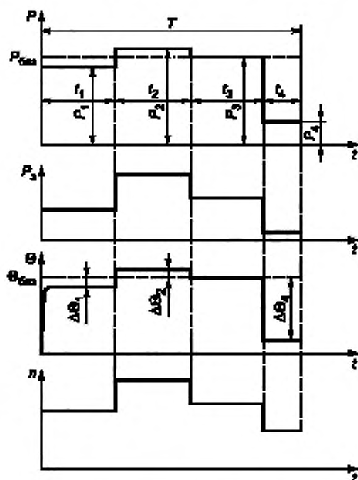
P — нагрузка, P_{\text{баз}} — базовая нагрузка в соответствии с типовым режимом S1, P_{1,2,3,4} — постоянная часть нагрузки внутри одного цикла нагрузки; P_z — электрические потери, \theta — температура, \theta_{\text{баз}} — температура при базовой нагрузке P_{\text{баз}} ; t — время, t_{1,2,3,4} — время работы с постоянной нагрузкой внутри цикла нагрузки; T — время одного цикла нагрузки, \Delta\theta_{1,2,3,4} — разница между превышением температуры обмоток при каждой из различных нагрузок внутри одного цикла и превышением температуры при базовой нагрузке в режиме S1; n — частота вращения
