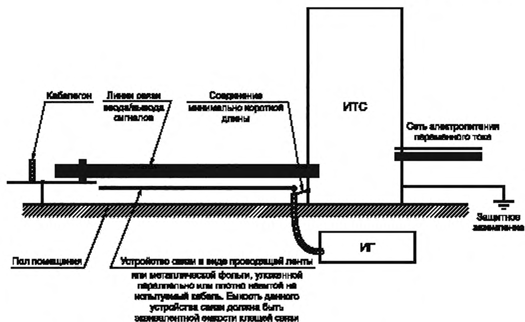
Рисунок 13 — Пример установки для испытаний ТС на месте эксплуатации с подачей НИП на порты ввода/вывода сигналов без использования емкостных клемм связи
