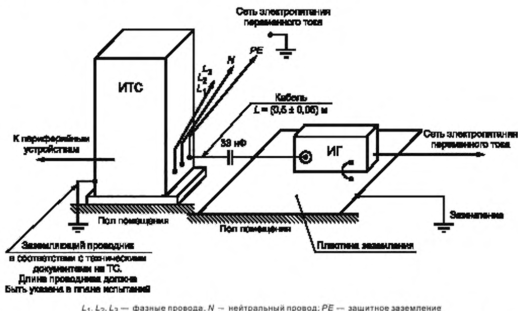
Рисунок 11 — Пример установки для испытаний стационарного напольного ТС на месте эксплуатации с подачей НИП на порты электропитания переменного и постоянного тока и порт защитного заземления
