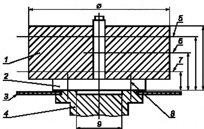
1 — ротор; 2 — переходник; 3 — уголок; 4 — шпиндель; 5 — верхняя плоскость коррекции; 6 — плоскость центра масс; 7 — нижняя плоскость коррекции; 8 — крепежные отверстия для переходника; 9 — центрирующий выступ (диаметр)
