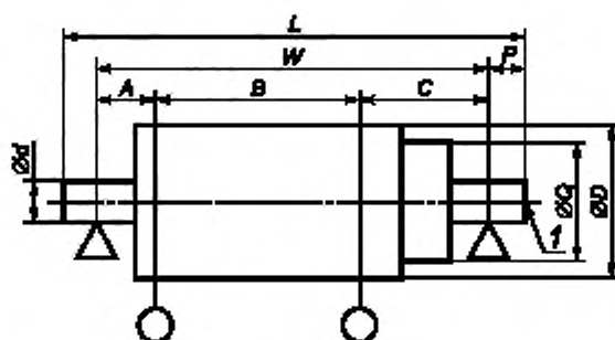
Рисунок А.2 — Нагрузки на опоры
