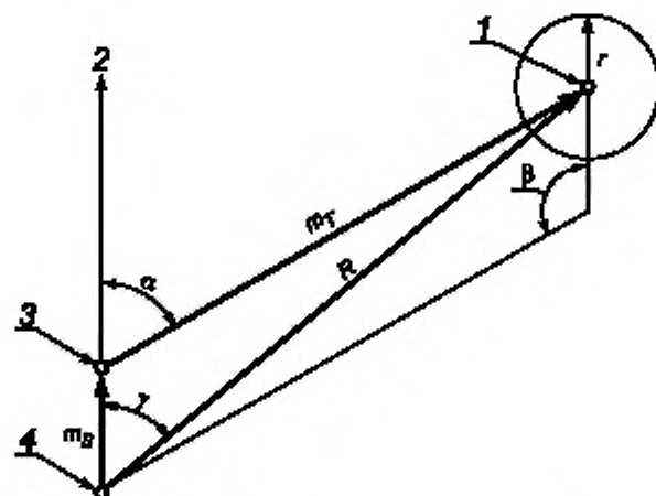
1 — центр окружностей-изолиний URR; 2 — ось полярной системы координат (0°); 3 — центр базовой окружности (геометрического места центров окружностей-изолиний URR); 4 — центр диаграммы
