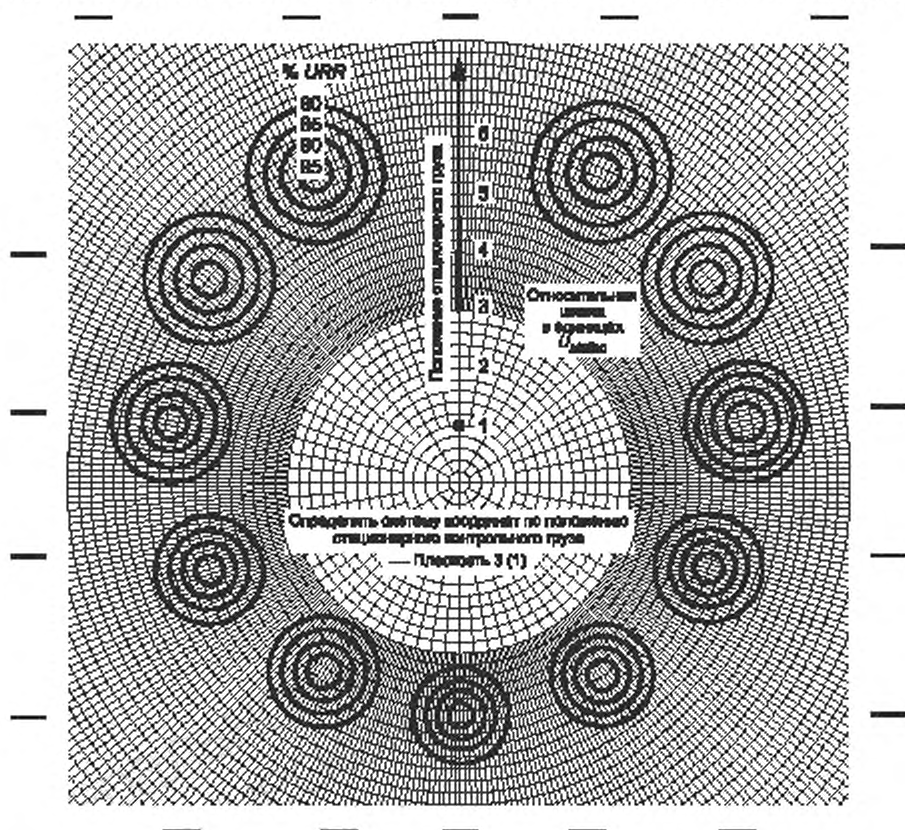
Рисунок 15 — Диаграмма оценки URR для испытания в одной плоскости
