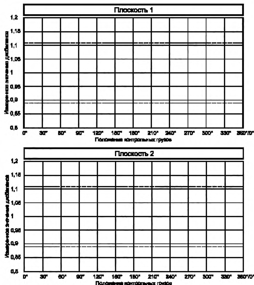
Рисунок 11 — График для оценки минимально достижимого остаточного дисбаланса
