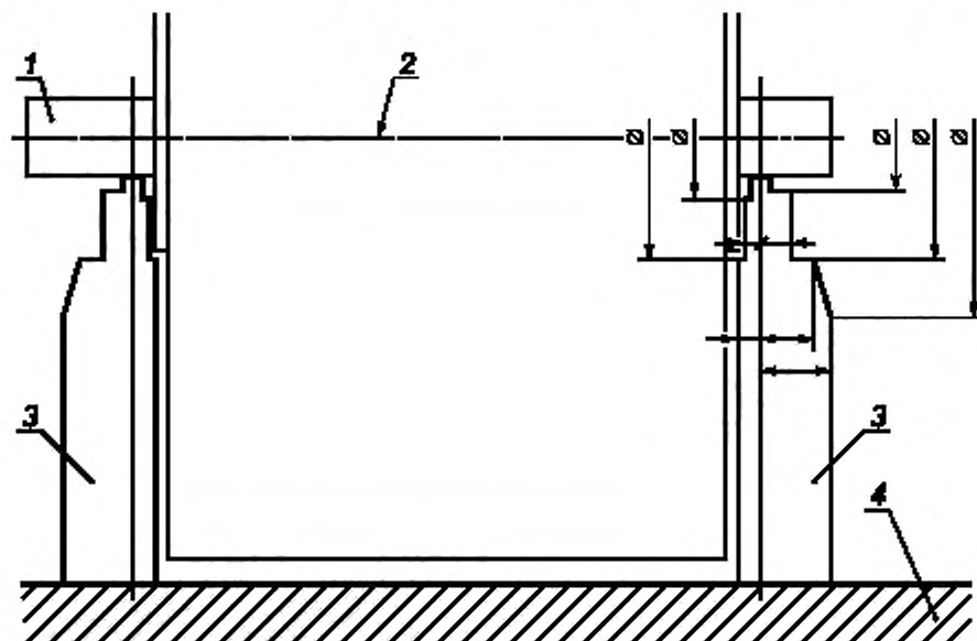
1 — вал; 2 — ротор; 3 — стойки; 4 — станина
