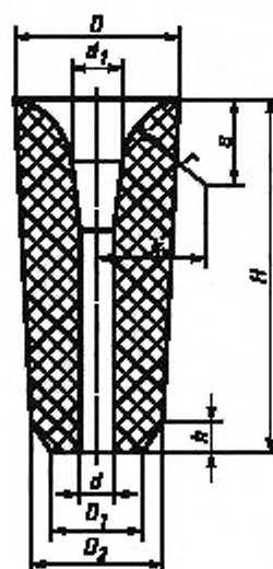
Рисунок 4 — Стакан-дозатор номеров 9—12, 15, 16, 18
