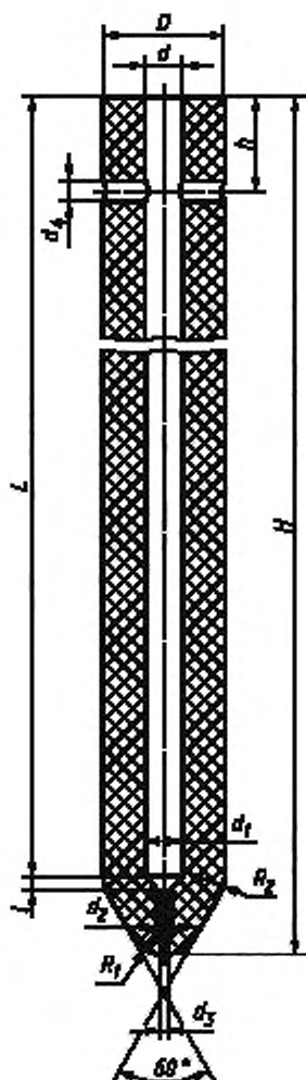
Рисунок 2 — Стопор-моноблок номеров 3,4
