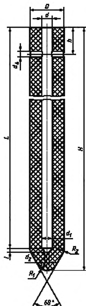
Рисунок 3 — Стопор-моноблок номеров 2,5
