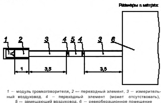
Рисунок 1 — Испытательная установка
