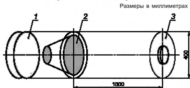
Рисунок 1 — Испытательная установка
