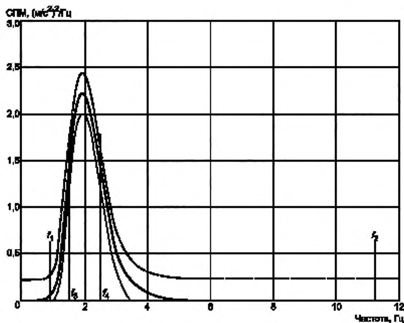
Рисунок 2 — СМН для спектрального класса ЕМ 1 (самосвал с жесткой или шарнирно-сочлененной рамой снаряженной массой более 4500 кг)
