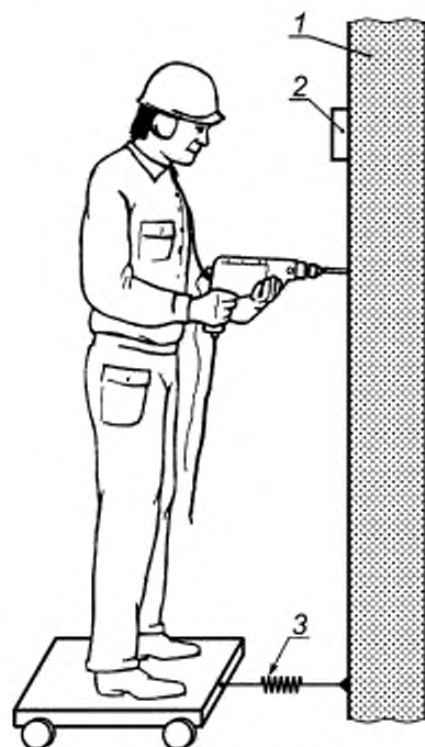
1 — бетонная стена; 2 — устройство считывания силы нажатия; 3 — динамометр
