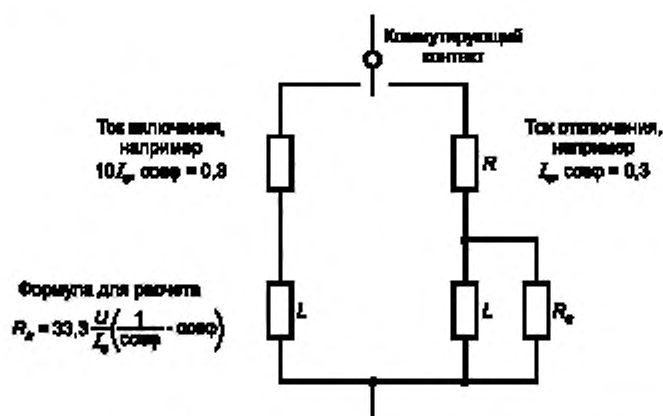
Рисунок 7 — Схема нагрузки L_x для условий испытаний, требующих различных значений токов включения и отключения и/или коэффициентов мощности (постоянной времени)
