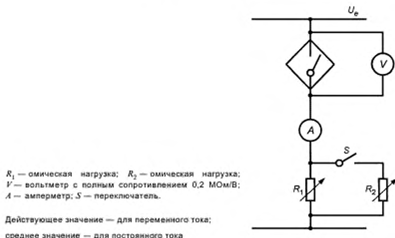
Рисунок Н.2 — Схема для проверки падения напряжения, минимального рабочего тока и тока в отключенном состоянии элемента (см. Н.8.2, Н.8.3 и Н.8.4)
