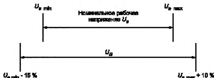
Рисунок Н.1 — Соотношение между U_r и U_B
