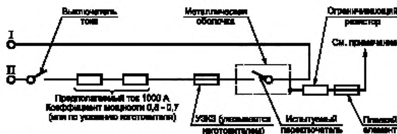
Рисунок 8 — Испытательная схема при проверке условного тока короткого замыкания
