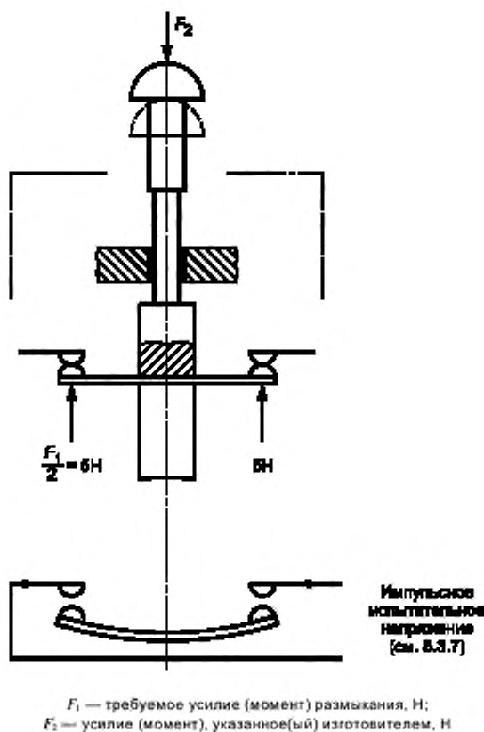
Рисунок К.1 — Проверка прочности механизма передачи усилия
