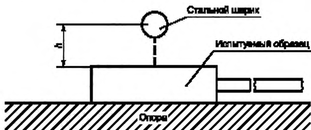
Рисунок F.2 — Испытательная установка
