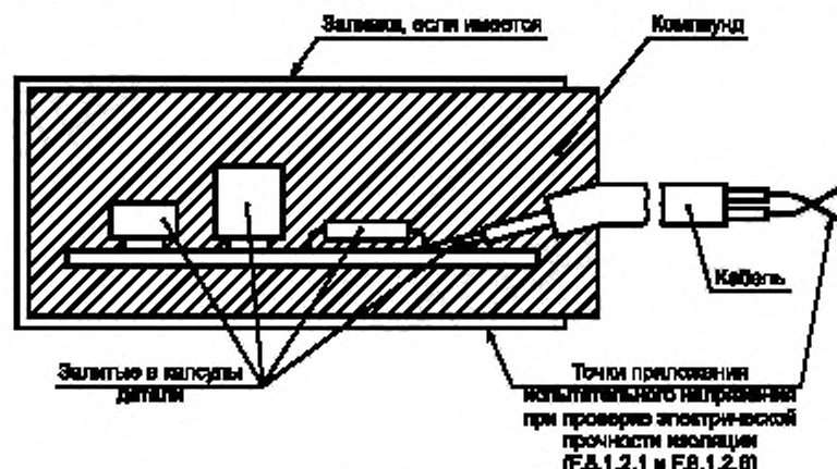
Рисунок F.1 — Изоляция заливкой в капсулы
