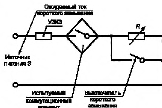
Рисунок Н.3 — Схема испытания на короткое замыкание
