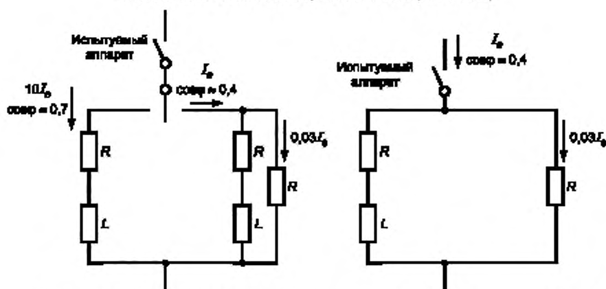
Рисунок С.1 — Полная схема (см. С.3.2.1)
