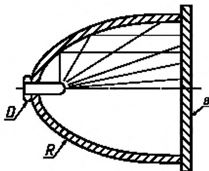
D — излучатель; R — рефлектор; B — фотоприемник
