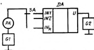
DA — измеряемая микросхема; IN1, IN2, \dots, INr — управляющие входы; U — вывод питания; G1, G2 — источники постоянного напряжения; SA — переключатель; PA — измеритель тока
