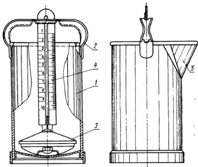
1 — корпус; 2 — ручка; 3 — поплавок; 4 — шкальная пластина; 5 — носик
