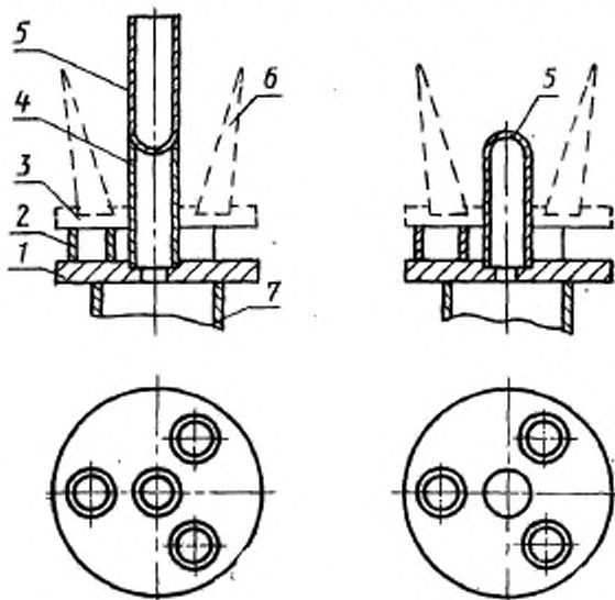
1 — подставка под модель «черное тело»; 2 — опорные конусы; 3 — подставка с испытательными конусами; 4 — опорная корончатая трубка; 5 — модель «черное тело»; 6 — испытательные конусы; 7 — огнеупорная труба механического приспособления печи
