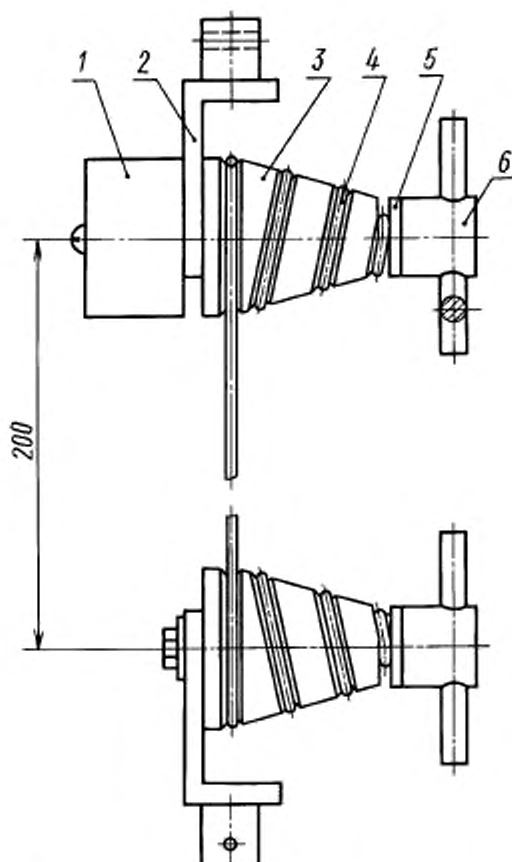
1 — противовес; 2 — корпус; 3 — улитка; 4 — образец провода; 5 — шайба; 6 — зажим
