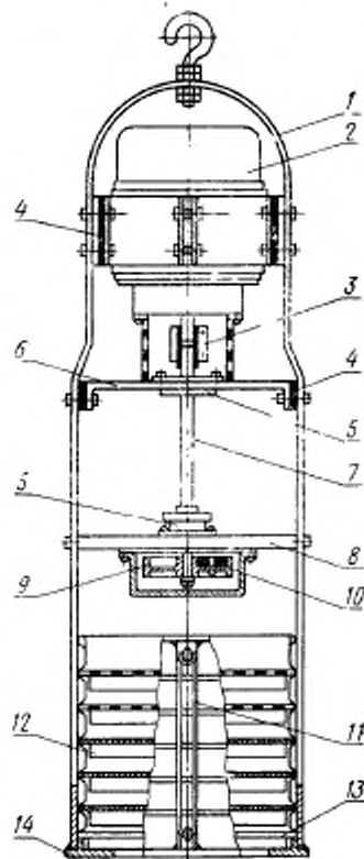
1—рама; 2—электромотор; 3—мягкая муфта; 4—резиновые прокладки; 5—шарики-подшипники; 6—верхняя площадка; 7—неуравновешенный валок вибратора; 8—площадка вибратора; 9—тарелка рамы; 10—груз; 11—резиновые кольца; 12—сито; 13—поддон; 14—тарелка рамы.
