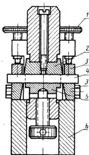
1 — винт; 2 — нож; 3 — опоры; 4 — образец; 5 — опорная планка; 6 — корпус
