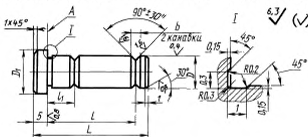
Размеры, мм
