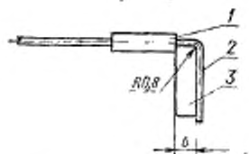
1 — изделие; 2 — вывод после изгиба; 3 — металлическая пластина
