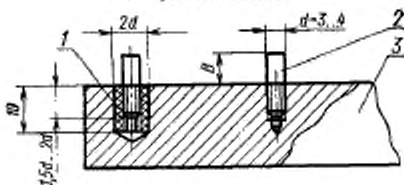
1 — изоляционная втулка; 2 — стойка; 3 — приспособление Черт. 2
