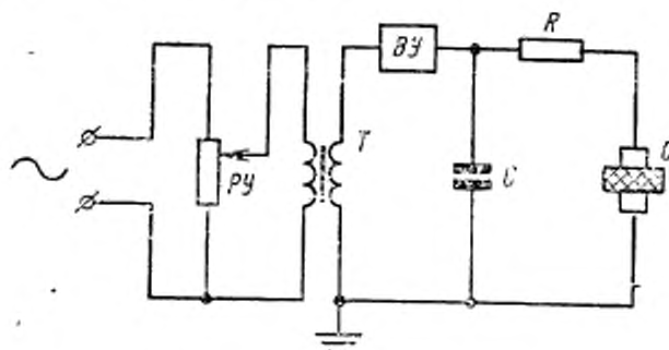
Т—высоковольтный испытательный трансформатор; R—защитное сопротивление; РУ—устройство, позволяющее осуществить плавный подъем напряжения на образце; О—образец; С—конденсатор; ВУ—выпрямительное устройство
