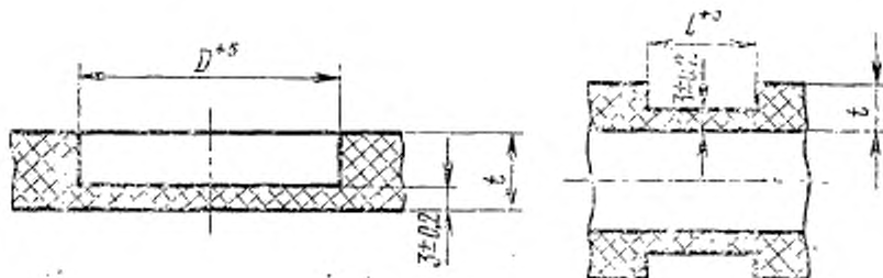
Трубчатый или цилиндрический образец
