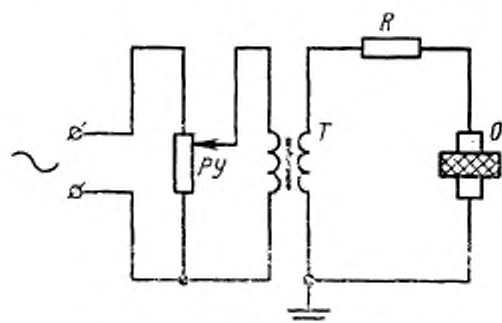
Т—высоковольтный испытательный трансформатор; R—защитное сопротивление; ПУ—устройство, позволяющее осуществлять подъем напряжения на образце; О—образец с электродами
