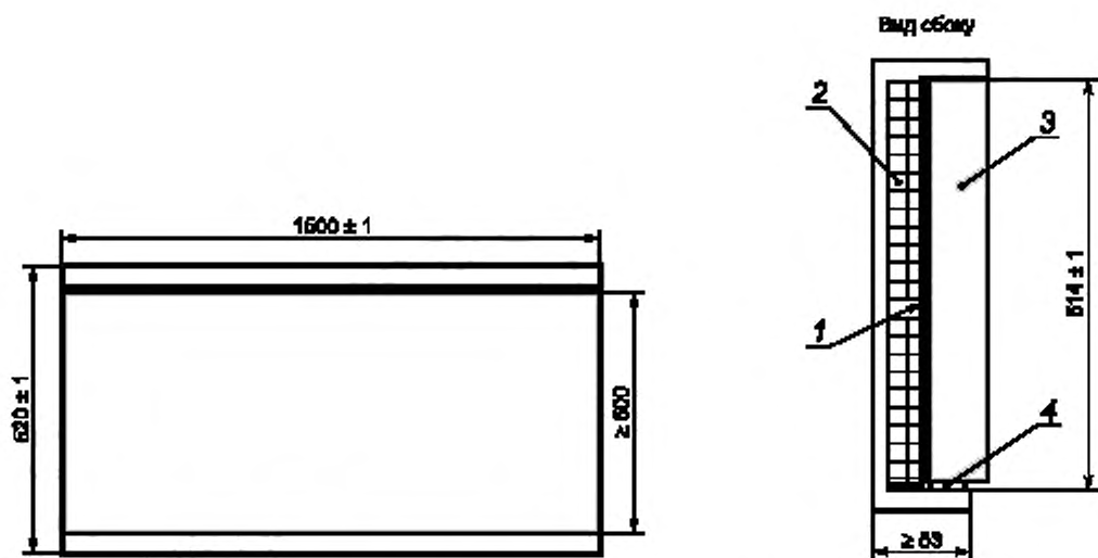
Рисунок 5 — Схема задней панели (вид спереди)
