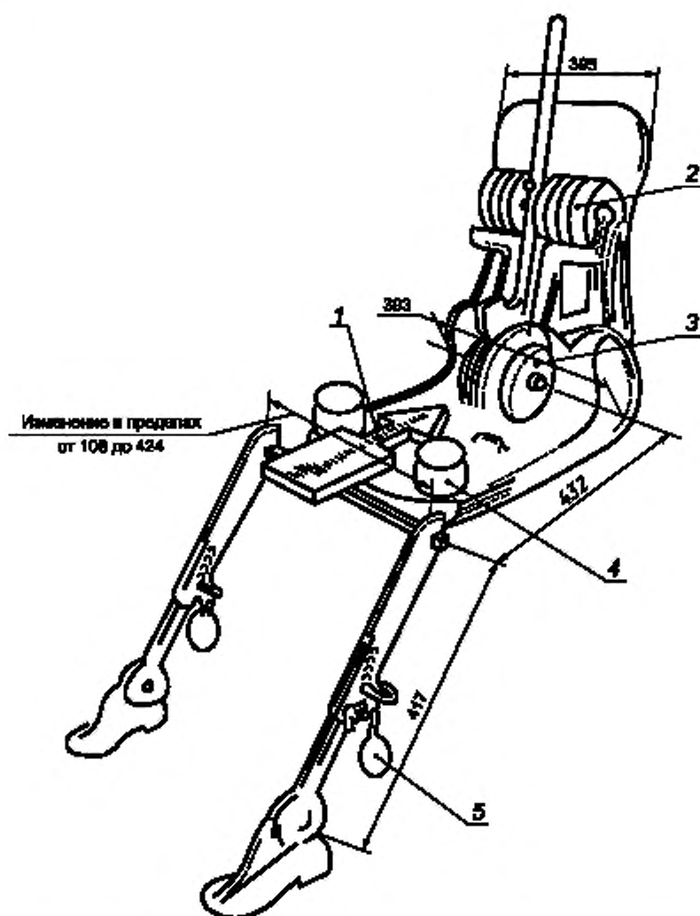
1 — направление и точка приложения нагрузки; 2 — спинные грузы; 3 — сидельные грузы; 4 — набедренные грузы; 5 — ножные грузы
