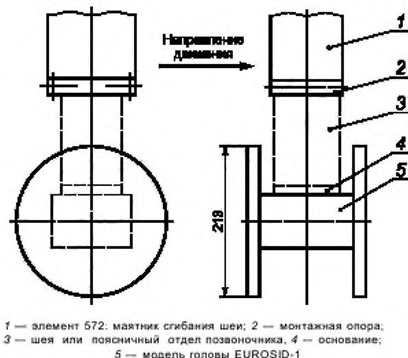
Рисунок 4 — Установка для испытания шеи и поясничного отдела позвоночника
