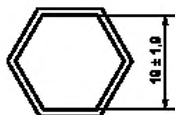
Рисунок 4 — Размер ячеек алюминиевой ячеистой конструкции
