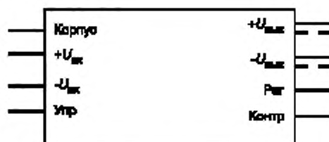
Рисунок Б.1 — Расположение выводов одноканальных СЭМ
