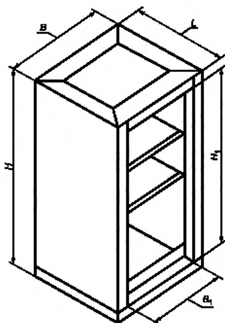
Рисунок 5 — Размеры корпусов СЭМ 3 на базе шкафа (стойки)
