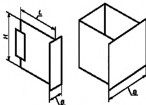
Рисунок 2 — Размеры корпусов СЭМ 1
