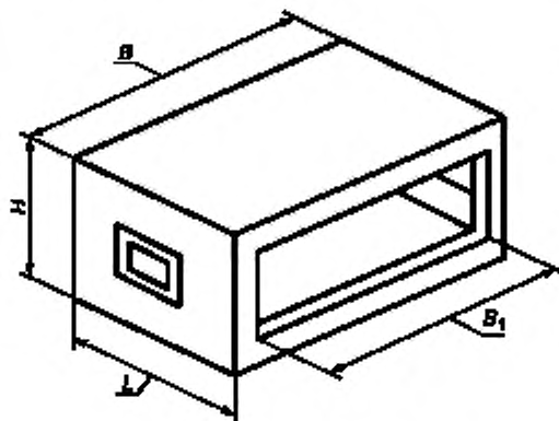
Рисунок 4 — Размеры корпусов СЭМ 3 на базе моноблока
