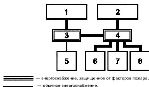
Схема энергоснабжения лифтов для пожарных
