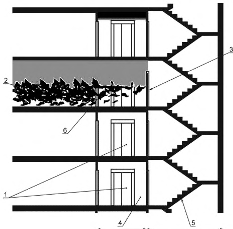
1 — лифт для пожарных; 2 — этаж пожара; 3 — огнестойкая дверь лифтового холла; 4 — пожарозащищенный лифтовой холл; 5 — пестница (путь эвакуации); 6 — разрушенная огнестойкая дверь или стена лифтового холла
