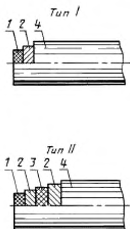
Рукава Z с оплетками из латунированной проволоки
