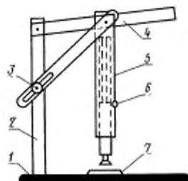
1 — основание; 2 — стойка; 3 — установочный винт; 4 — рычаг; 5 — гильза с винтовой пружиной; 6 — контрольная отметка; 7 — пластинка для испытания
