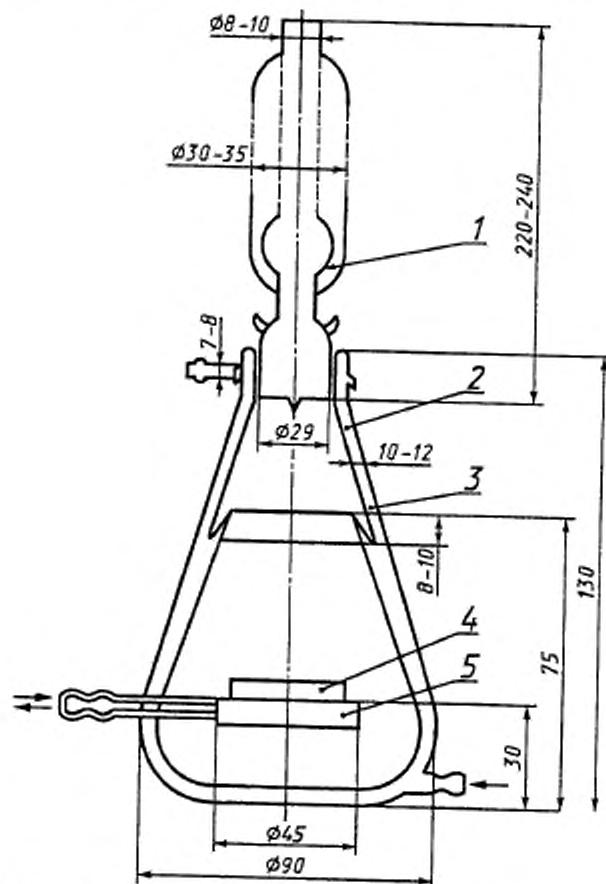
Аппарат для определения коррозионной активности бензинов
