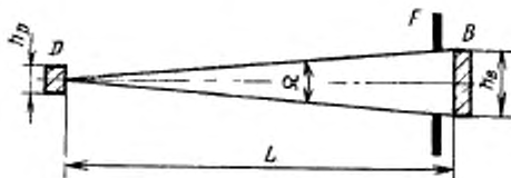
D—излучатель; h_D —размер излучающей поверхности, перпендикулярной к геометрической оси фотоприемника; \alpha —телесный угол излучения; L—расстояние от излучателя до приемной площадки фотоприемника; F—диаграмма; B—фотоприемник; h_B —размер освещенного участка
