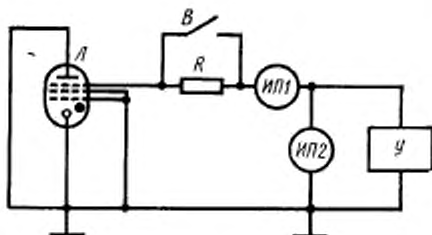
R — резистор; В — выключатель; ИП1 — измеритель тока; ИП2 — измеритель напряжения; Л — испытуемый тиратрон; У — регулируемый источник постоянного напряжения
