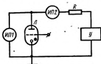
R — резистор; ИП1 — измеритель напряжения; ИП2 — измеритель тока; Л — испытуемый тиратрон (газотрон); У — регулируемый источник постоянного напряжения
