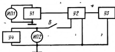
B —выключатель; ИП1 , ИП2 —измерители напряжения; У1 —регулируемый источник постоянного напряжения; У2 —устройство коммутации и испытуемый тиристор; У3 —осциллограф; У4 —генератор входных сигналов
