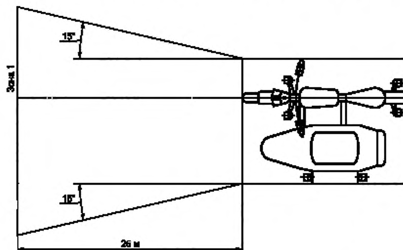
Рисунок В.1 — Видимость красного огня в направлении вперед (5.9.1)
