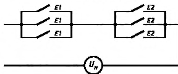
Схема включения главных контактов контакторов при испытании механической блокировки
