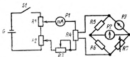
R5 , R6 , R7 — сопротивления плеч измерительного моста постоянного тока; P2 — нулевой указатель измерительного моста; P3 — поверженный гальванометр
