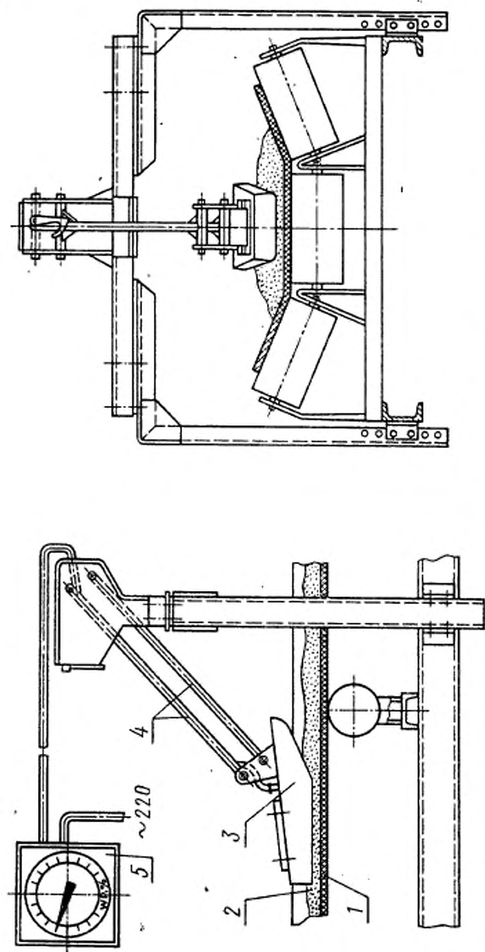
1—денотный конвейер; 2—поток угля; 3—измерительный преобразователь; 4—подвеска измерительного преобразователя; 5—регистрирующий прибор с электронным блоком.
